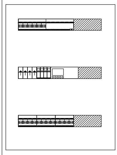
IMPIANTO FV SCUOLA MEDIA FABRICA: QUADRO FOTOVOLTAICO QUADRO DA PARETE IN PVC IP40 - 3X18 MODULI
