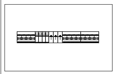
IMPIANTO FV SCUOLA MEDIA FABRICA: QUADRO DI CAMPO 2-4 QUADRO DA PARETE IN PVC IP55 - 1X18 MODULI
