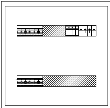
IMPIANTO FV SCUOLA MEDIA FABRICA: QUADRO GENERALE QUADRO DA PARETE IN PVC IP40 - 2X18 MODULI
