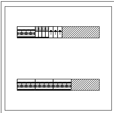
IMPIANTO FV SCUOLA MEDIA FABRICA: QUADRO DI CAMPO 1-3-5-6 QUADRO DA PARETE IN PVC IP55 - 2X18 MODULI
